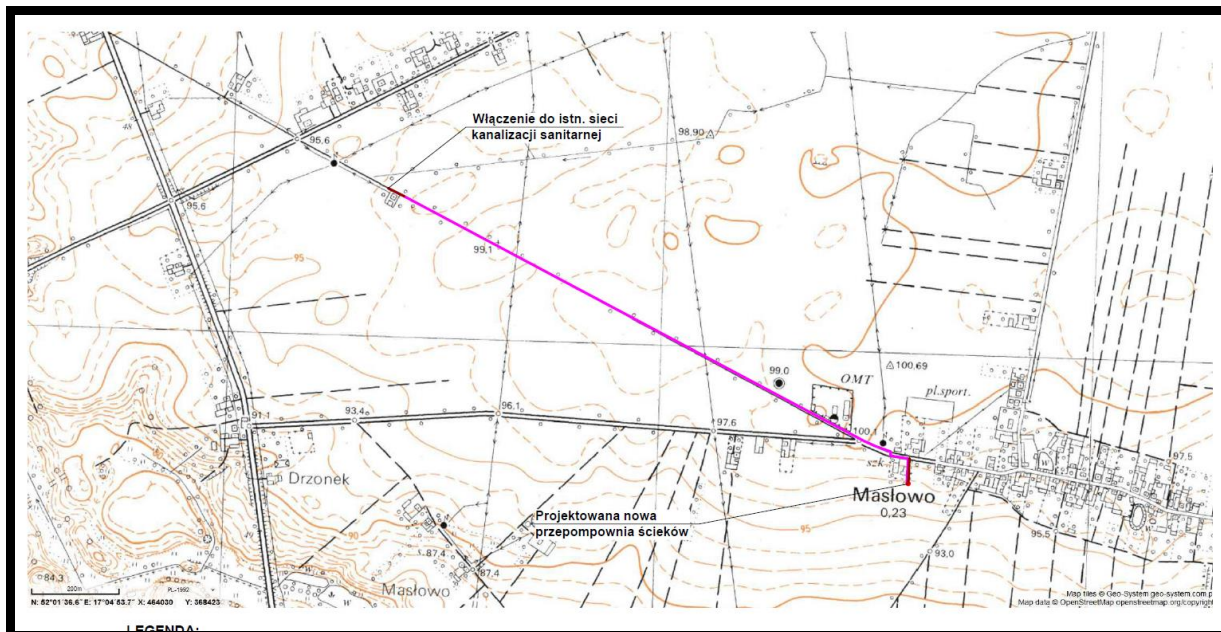
Położenie sieci kanalizacyjnej wraz z kolektorem i przepompownią ścieków w miejscowości Masłowo
